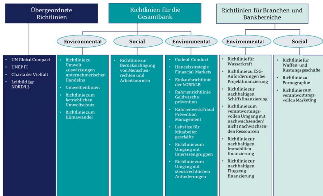
Abbildung 9: ESG Richtlinien
