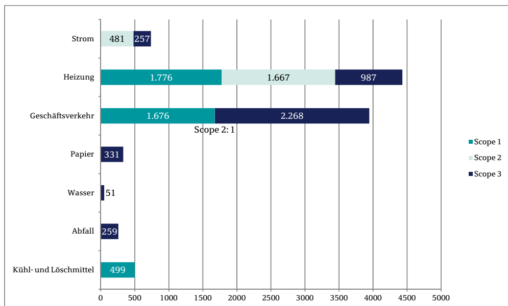
Abbildung 20: Ökologischer Fußabdruck
